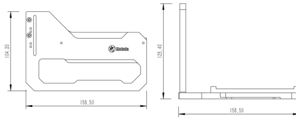
安装延长线尺寸图:
