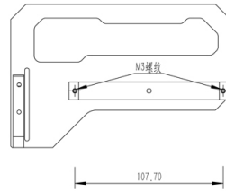
安装延长线尺寸图:
